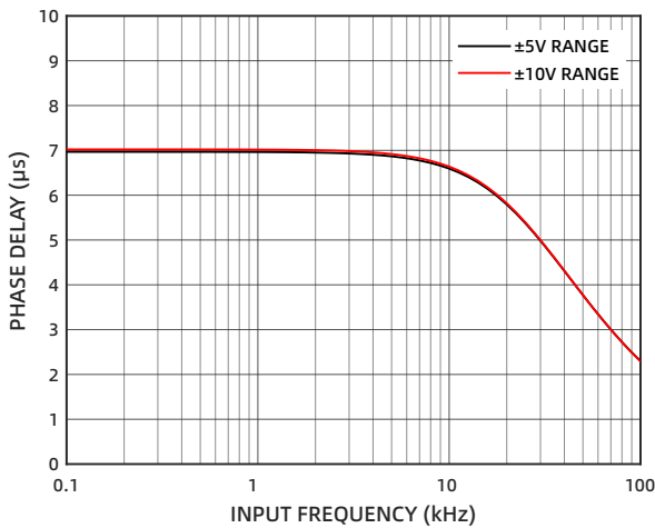
图 30 模拟抗混叠滤波器相频特性
