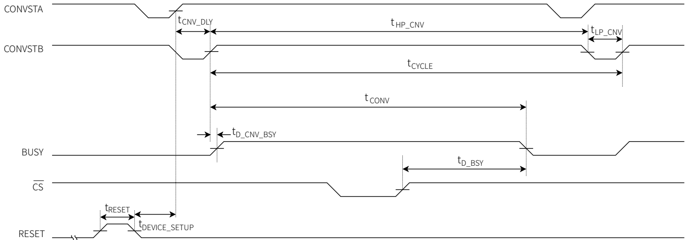
图 1 CONVST 时序-转换期间读取
