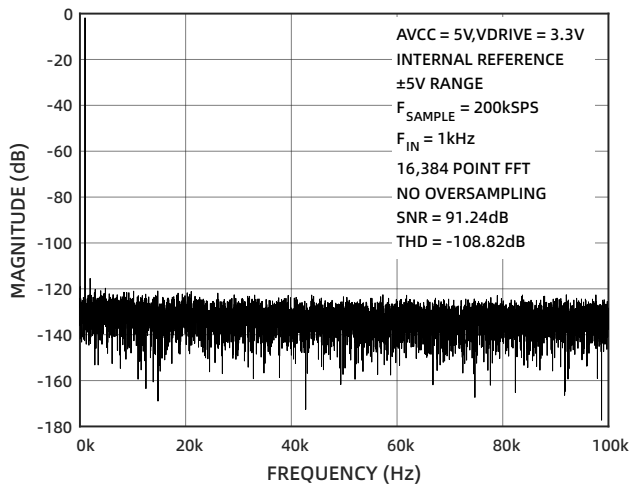
图 17 FFT (±5V)
