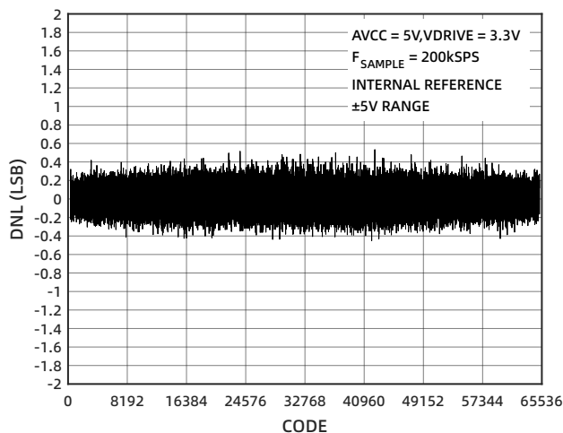
图 8 DNL (±5V)
