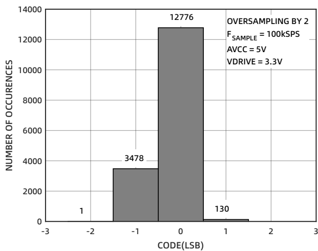
图 12 零输入直方图-OS×2
