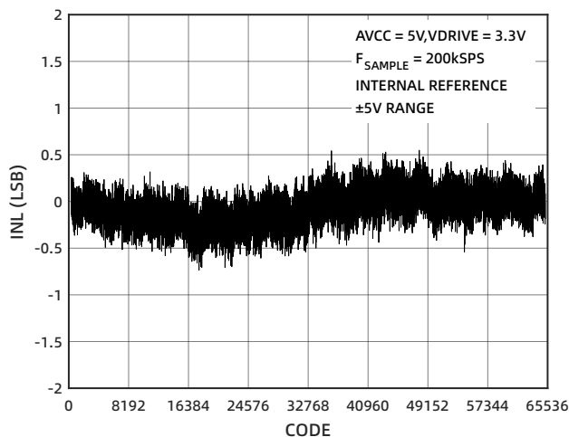
图 10 INL (±5V)
