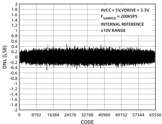
图 7 DNL (±10V)
