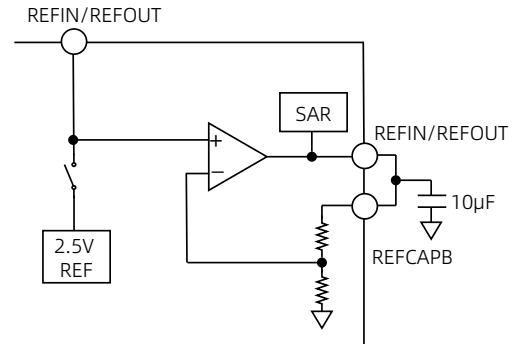
图 31 基准电压电路
