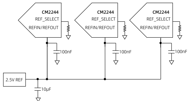
图 32 外部基准电压源驱动多个 CM2244
