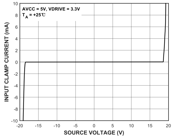
图 27 输入钳位电路 V-I 特性曲线
