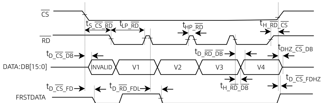
图 3 并行模式，独立的 \overline{CS} 和 \overline{RD} 脉冲
