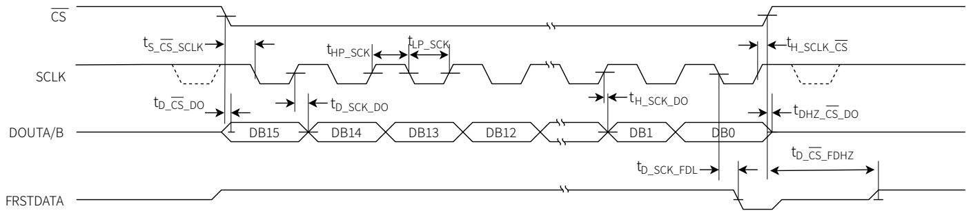
图 6 串行读取操作
