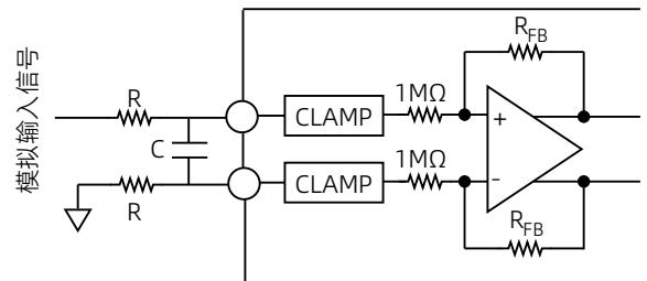
图 28 模拟输入端上输入电阻匹配
