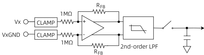
图 26 模拟输入电路
