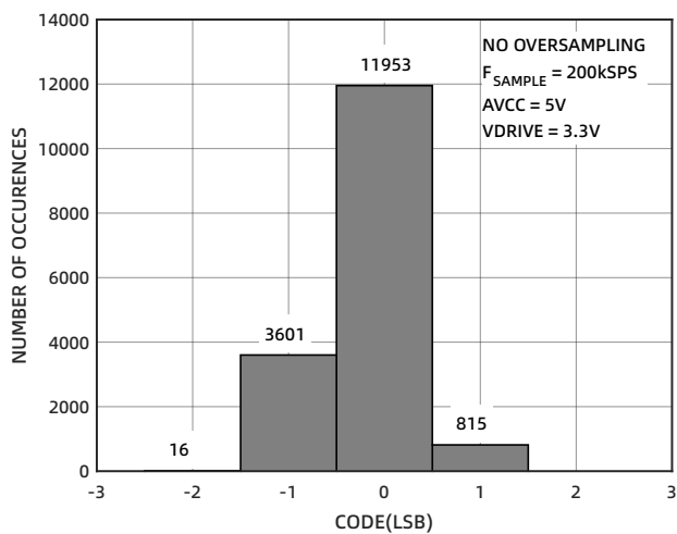
图 11 零输入直方图-无过采样
