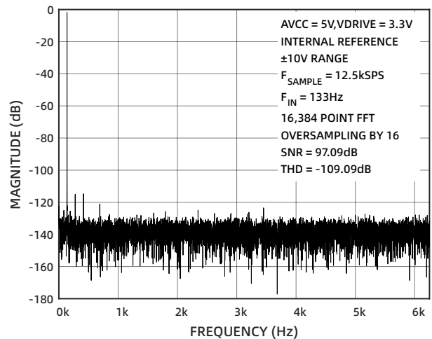
图 18 FFT 过采样 (±10V)
