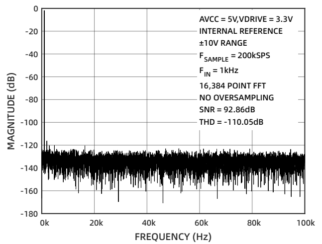
图 16 FFT 无过采样 (±10V)
