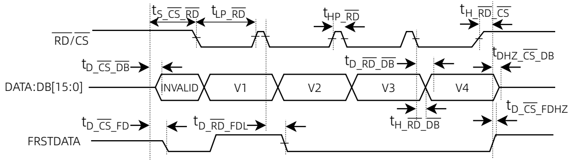
图 4 并行模式，CS和RD相连
