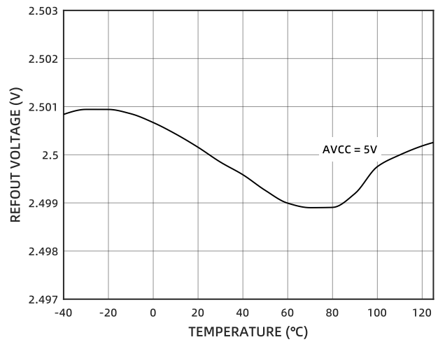
图 22 基准电压温漂
