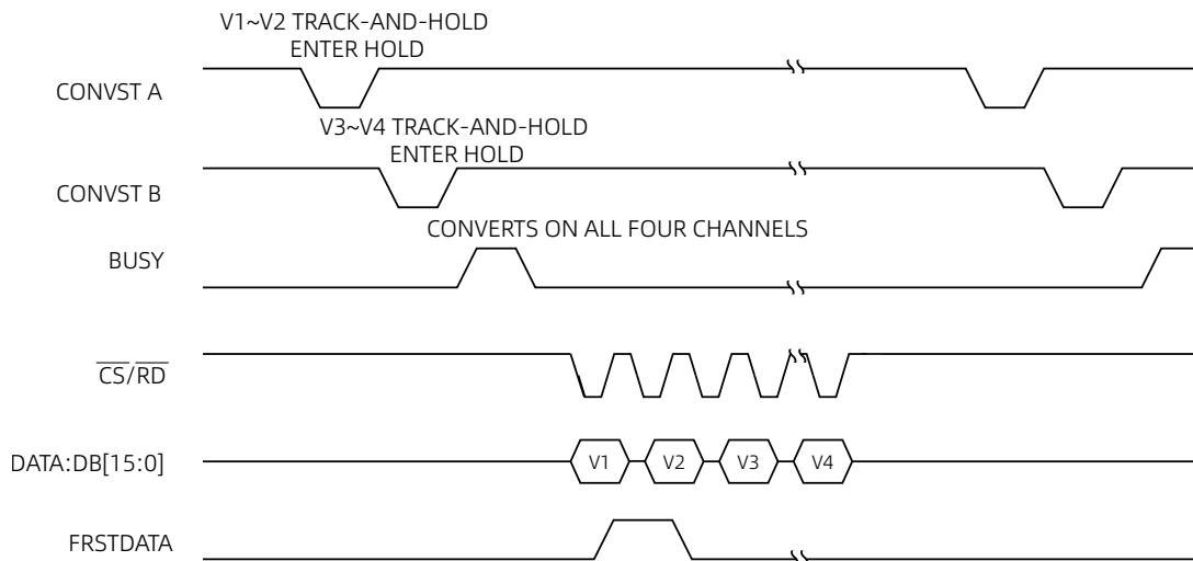
图 34 CONVSTA 和 CONVSTB 分别进行同步采样
