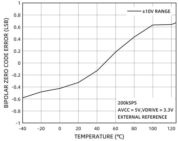
图 20 双极性 0 码误差的温度特性
