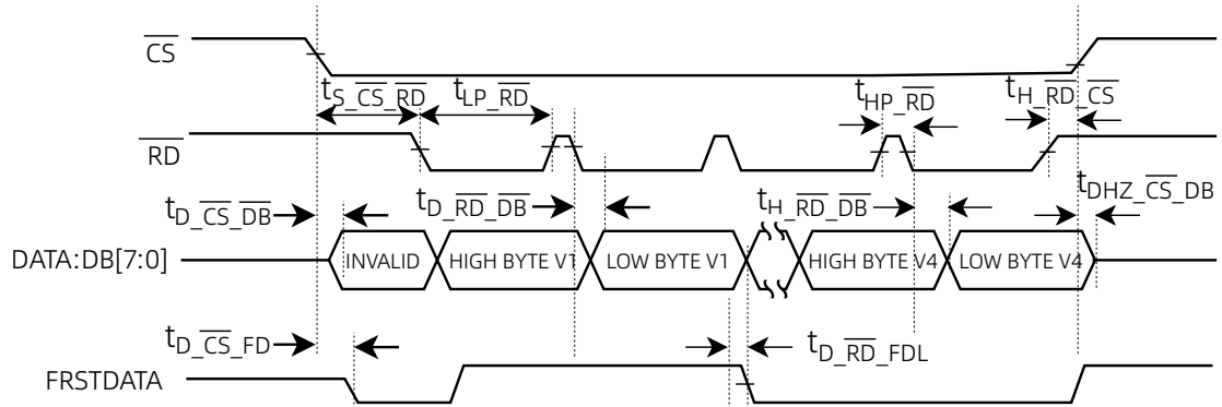
图 5 字节模式读取操作
