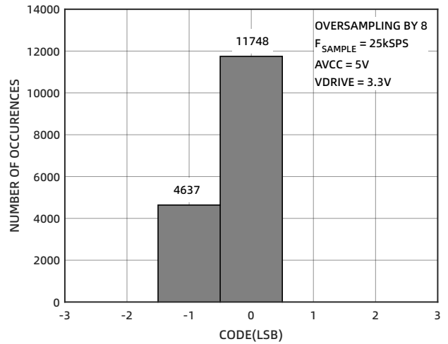
图 14 零输入直方图-OS×8
