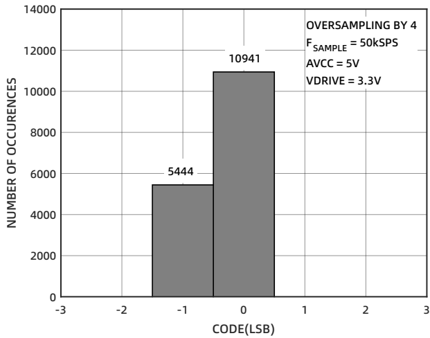
图 13 零输入直方图-OS×4
