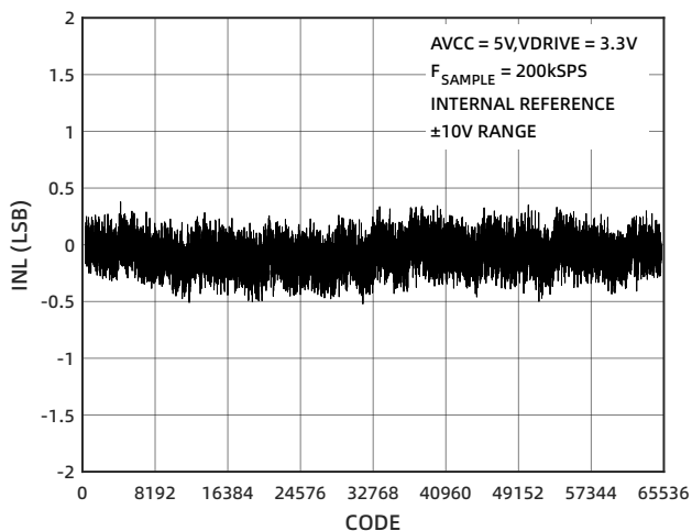
图 9 INL (±10V)
