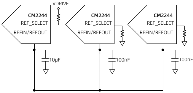
图 33 内部基准电压源驱动多个 CM2244
