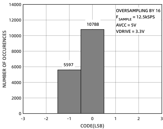
图 15 零输入直方图-OS×16
