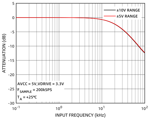
图 29 模拟抗混叠滤波器幅频特性
