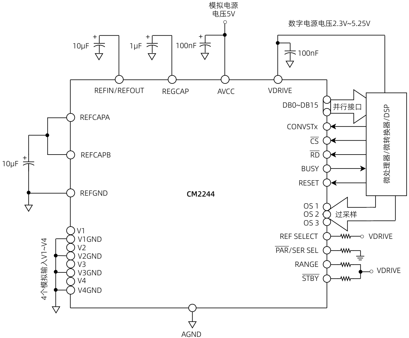
图 35 典型连接
