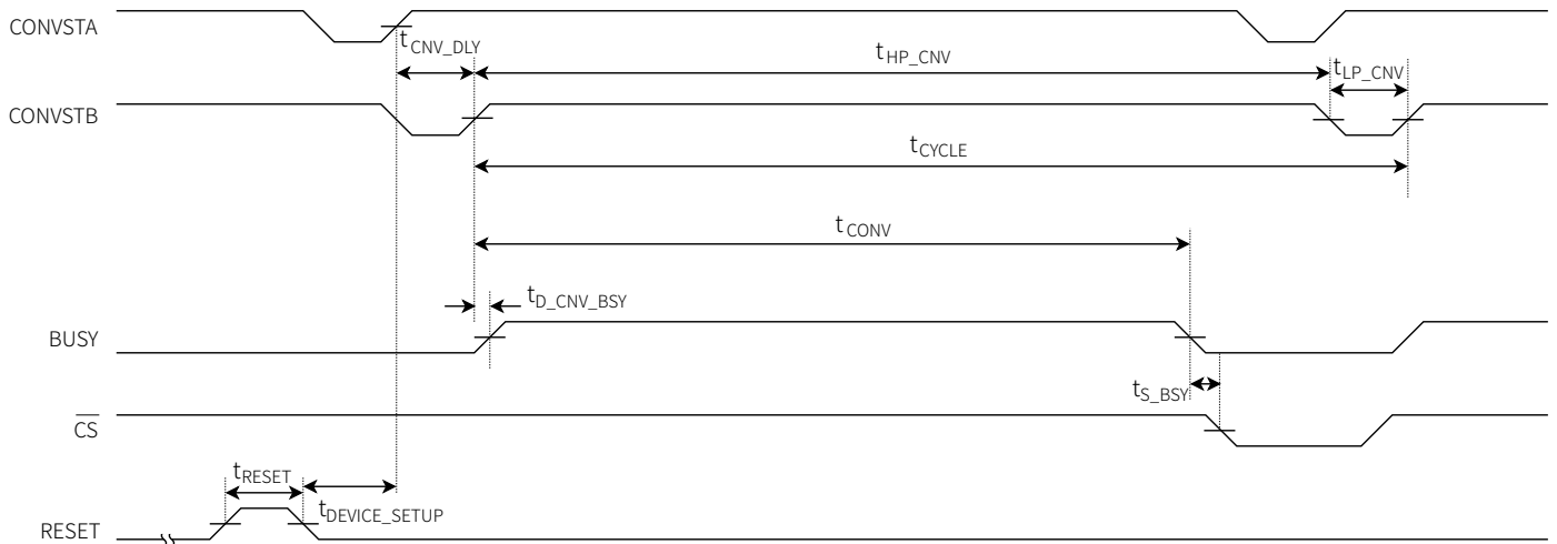
图 2 CONVST 时序-转换之后读取
