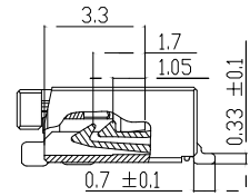
SECT: X-X 比例 4.000
