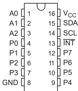
SOP16
