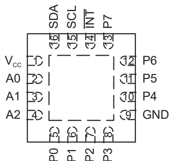
QFN16
