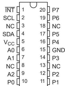
TSSOP20
