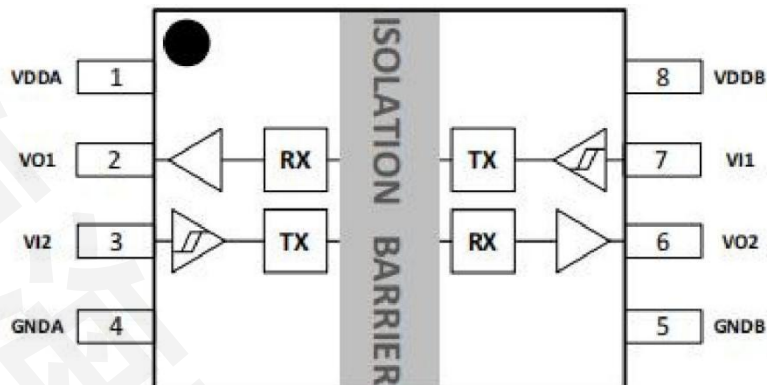
图 1. ADUM3201ARZ-HX/ADUM3201BRZ-HX/ADUM3201CRZ-HXSOP8(窄体)封装顶部视图
