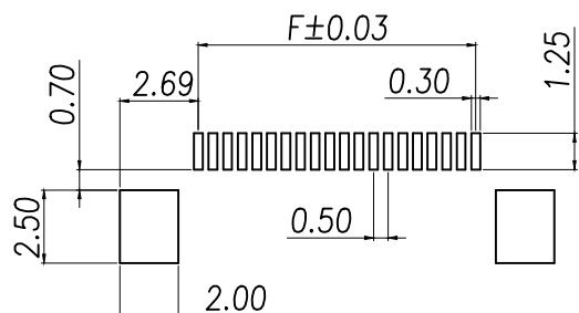
PCB 寸法 PCB Layout
