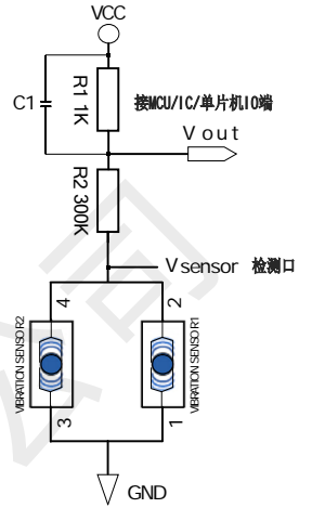
最可靠接法
