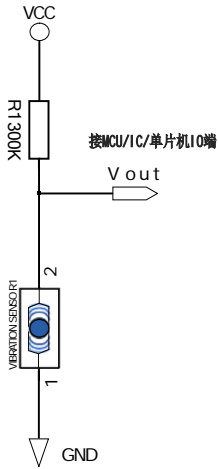
基本电路接法
