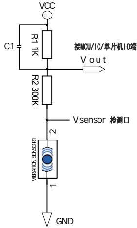
滤波电路接法
