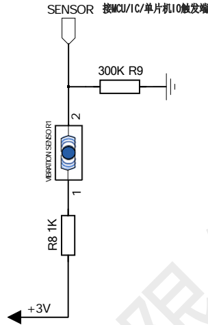
最省电接法
