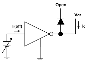
图3 I_{I(off)} 测试电路
