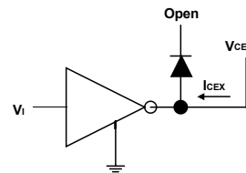
图2 I_{CEX} 测试电路
