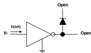
图 4 I_I 测试电路
