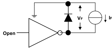
图8 V_R 测试电路
