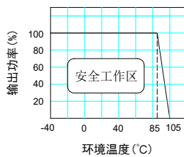
温度曲线图
