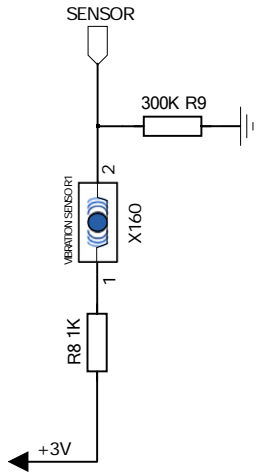
最省电接法
