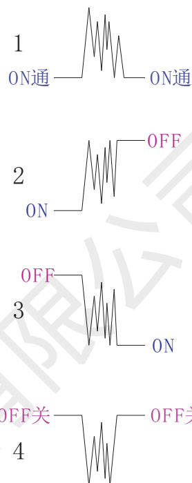
传感器信号形式: 4种表现
