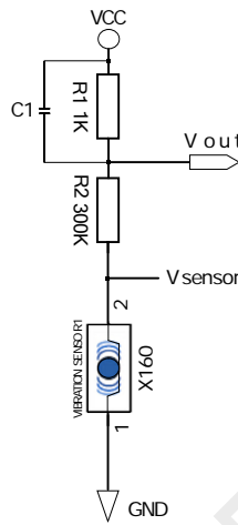
滤波电路接法
