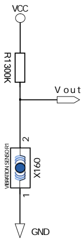
基本电路接法
