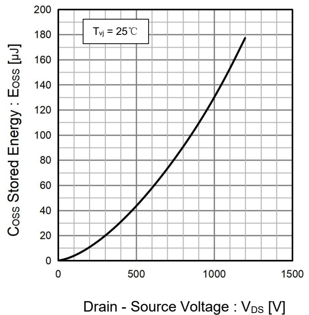
Fig.15 C_{oss} Stored Energy
