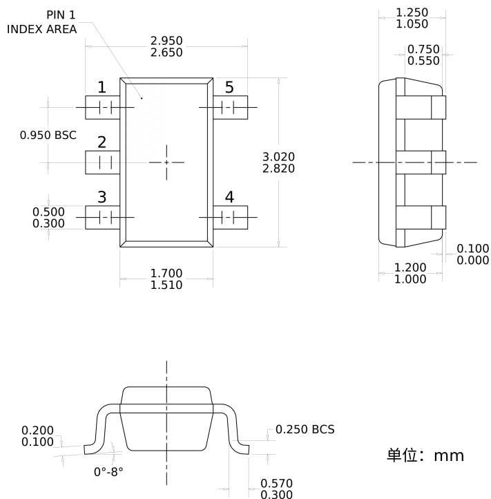
图 13: 封装 SOT23-5
