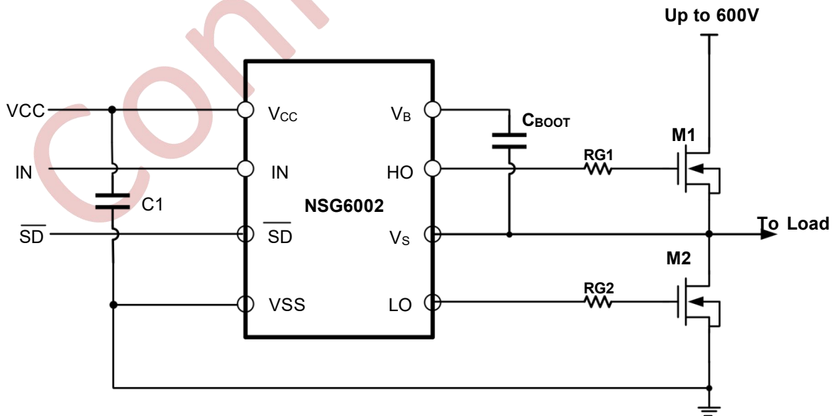
图 10-2 NSG6002 典型应用电路图
