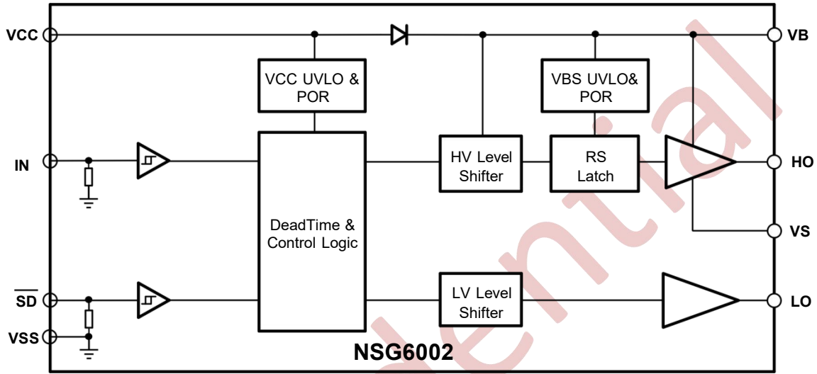
图 10-1 NSG6002 的功能框图
