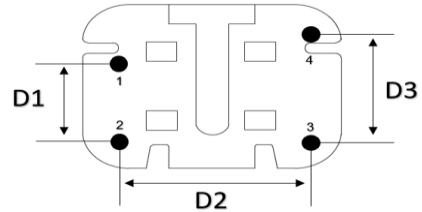
底视图 bottom view
