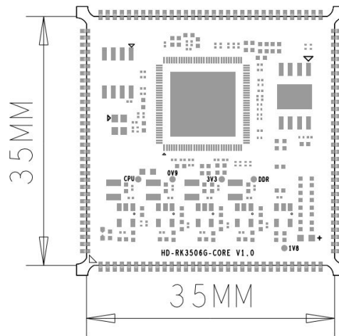
图 3 RK3506G 核心板尺寸图
