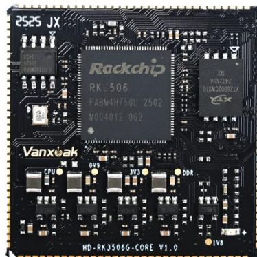
图 1 RK3506G 核心板
