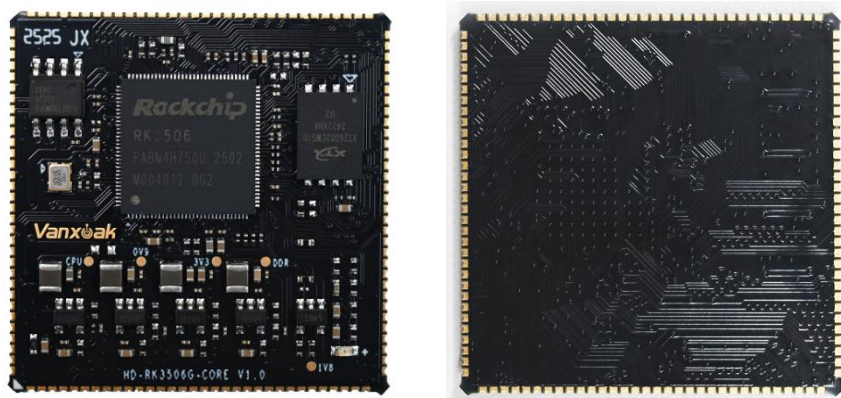
图 2 RK3506G 核心板顶底视图
