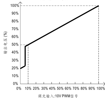
调光输入: 10V PWM信号
