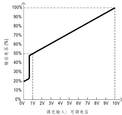
调光输入: 可调电压
