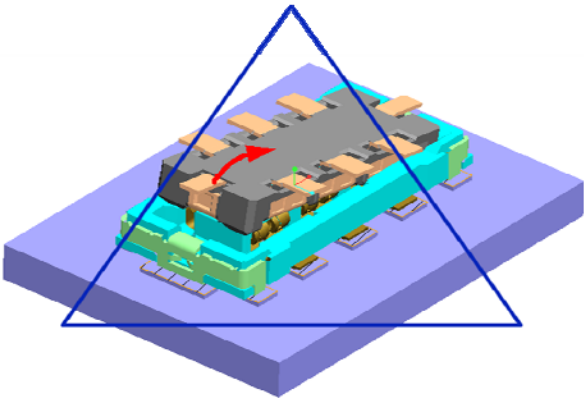
Slant releasing in “a” Direction (lengthways) 长方向的倾斜拔出
