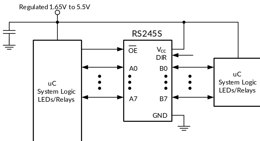
图 2. 典型应用原理图
