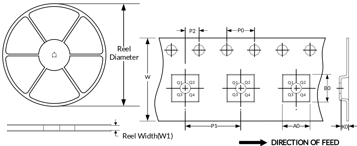
卷盘尺寸
