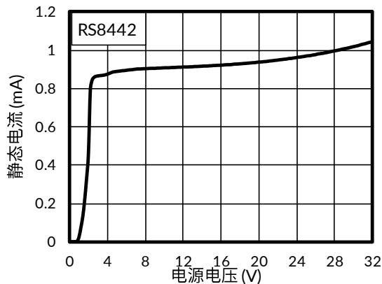
图 1. 静态电流与电源电压的关系
