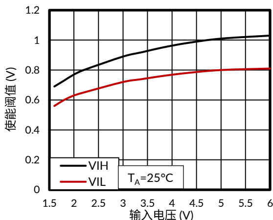
图 10. 使能阈值与输入电压的关系
