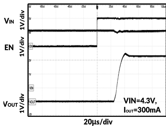
图 20. 开启时序
