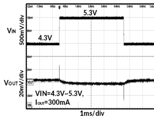
图 25. 线性瞬态响应 ( I_{OUT}=300mA )
