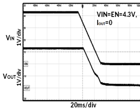
图 15. 下电时序
