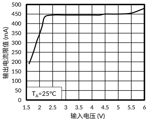
图 12. 输出电流限值与输入电压的关系
