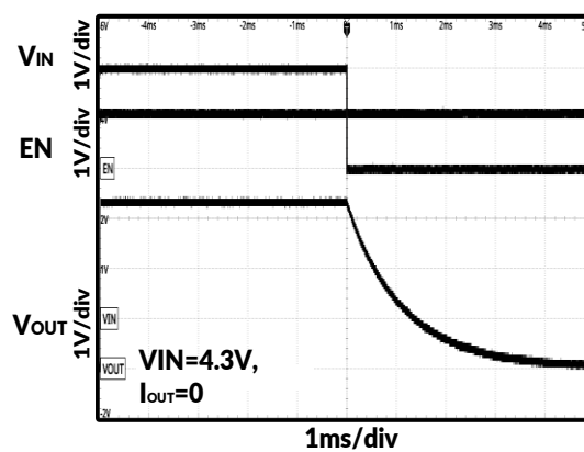
图 19. 关断时序
