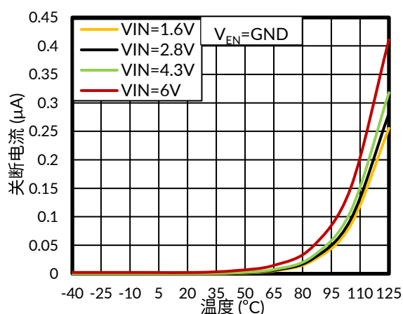
图 3. 关断电流与结温的关系
