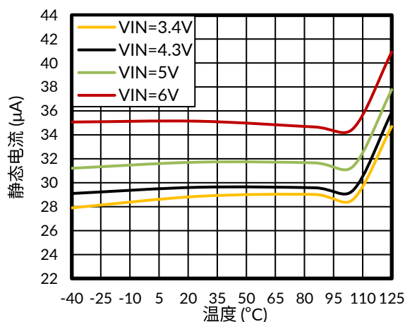
图 2. 静态电流与温度的关系
