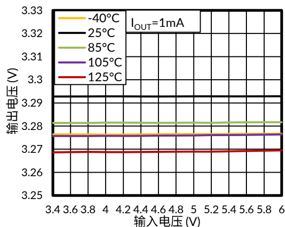
图 7. 线性调整率
