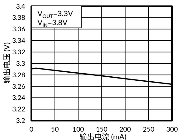
图 6. 负载调整率
