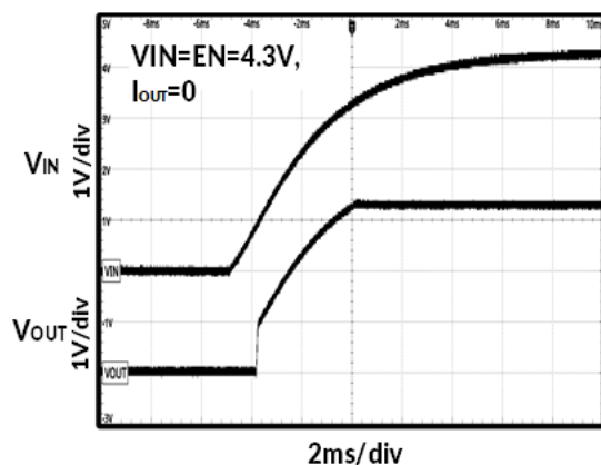
图 14. 上电时序
