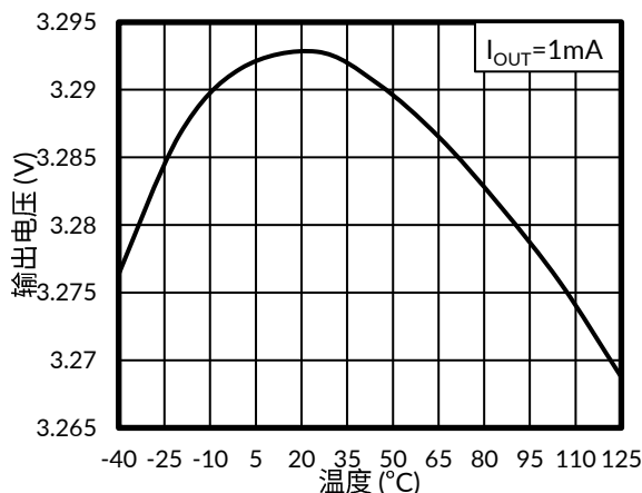
图 8. 输出电压与结温的关系
