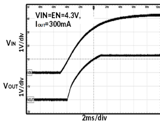
图 16. 上电时序
