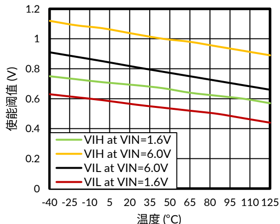
图 11. 使能阈值与结温的关系
