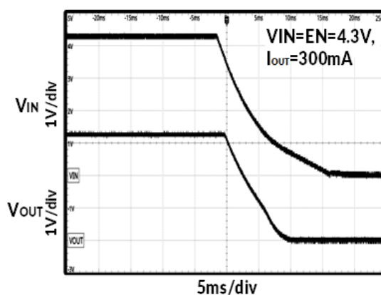
图 17. 下电时序
