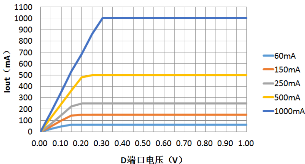
图 10.4.1 Hi12410W 恒流曲线
