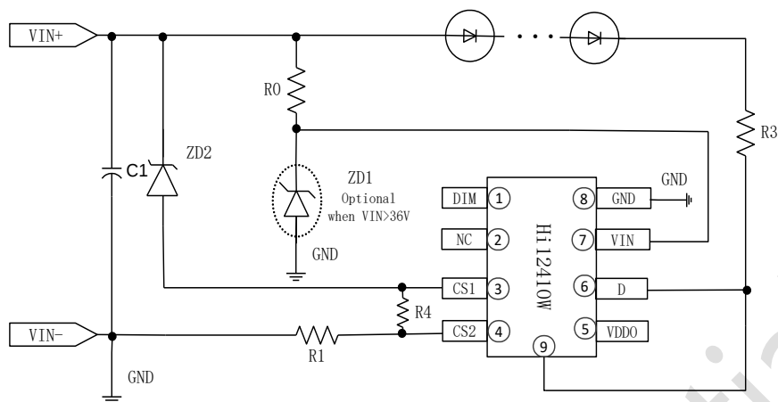
图 6.2 Hi12410W 过压保护电路
