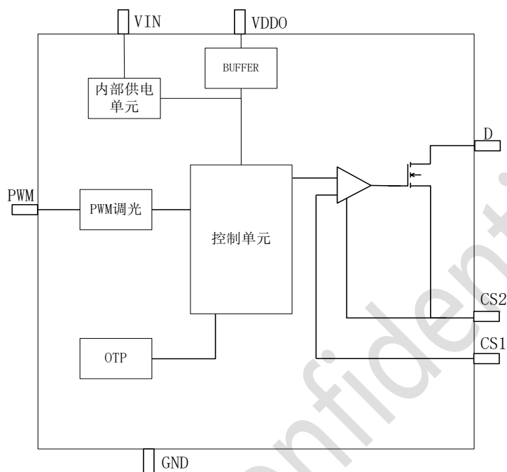
图 9 Hi12410W 结构框图
