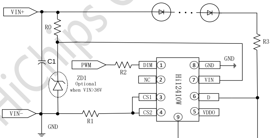
图 6.1 Hi12410W 应用电路
