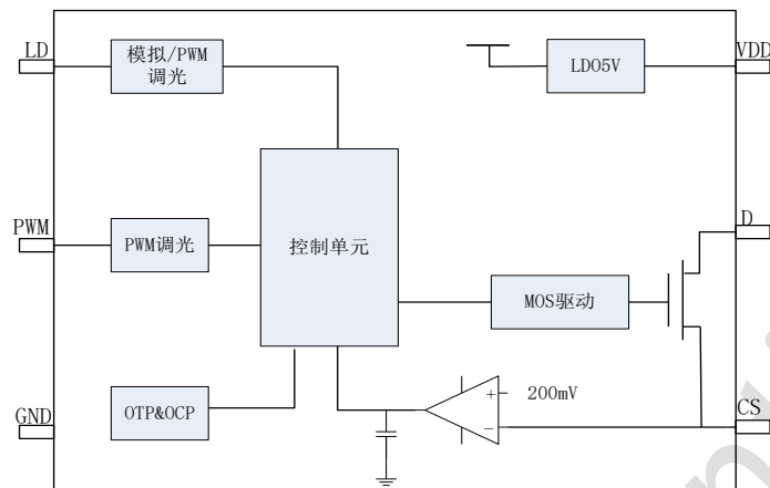
图 7.1 结构框图
