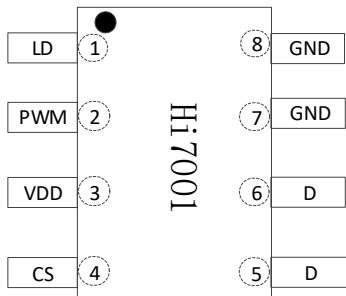
图 5.1 Hi7001 管脚图
