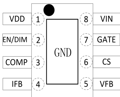
图 5.1 Hi6000A 管脚图
