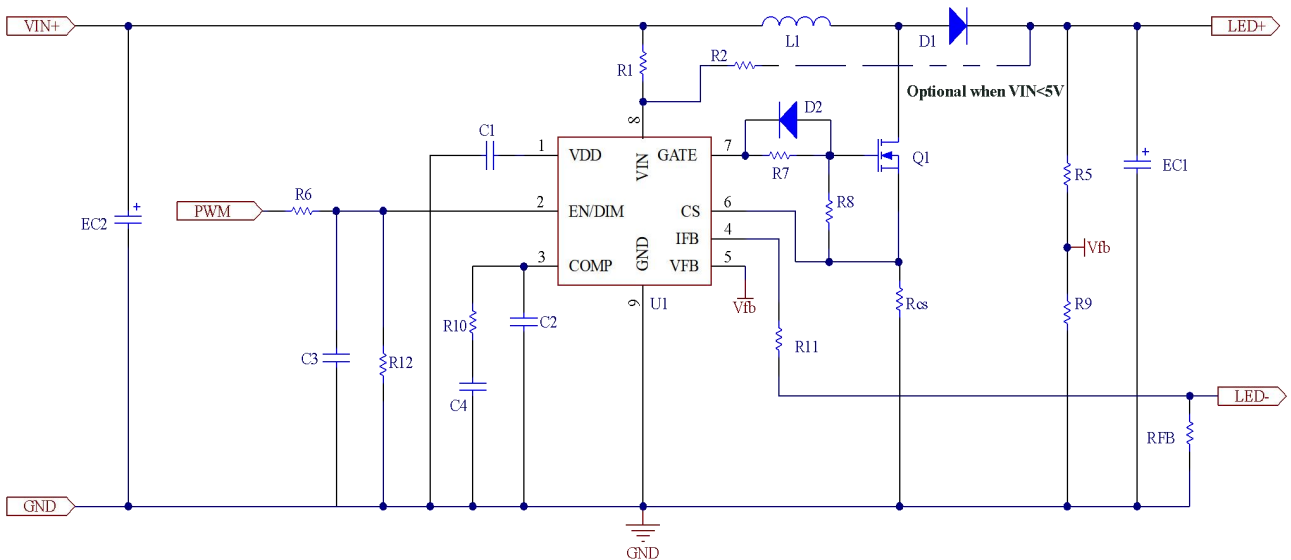
图 8.1 Hi6000A 典型应用电路
