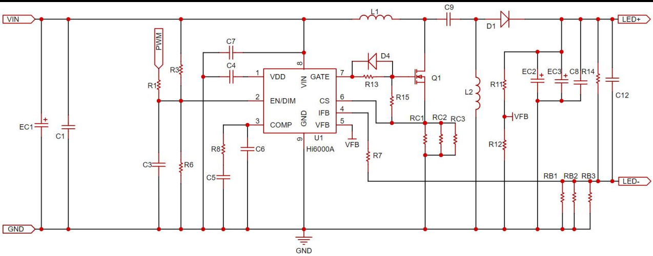
图 8.2 Hi6000A 升降压应用电路
