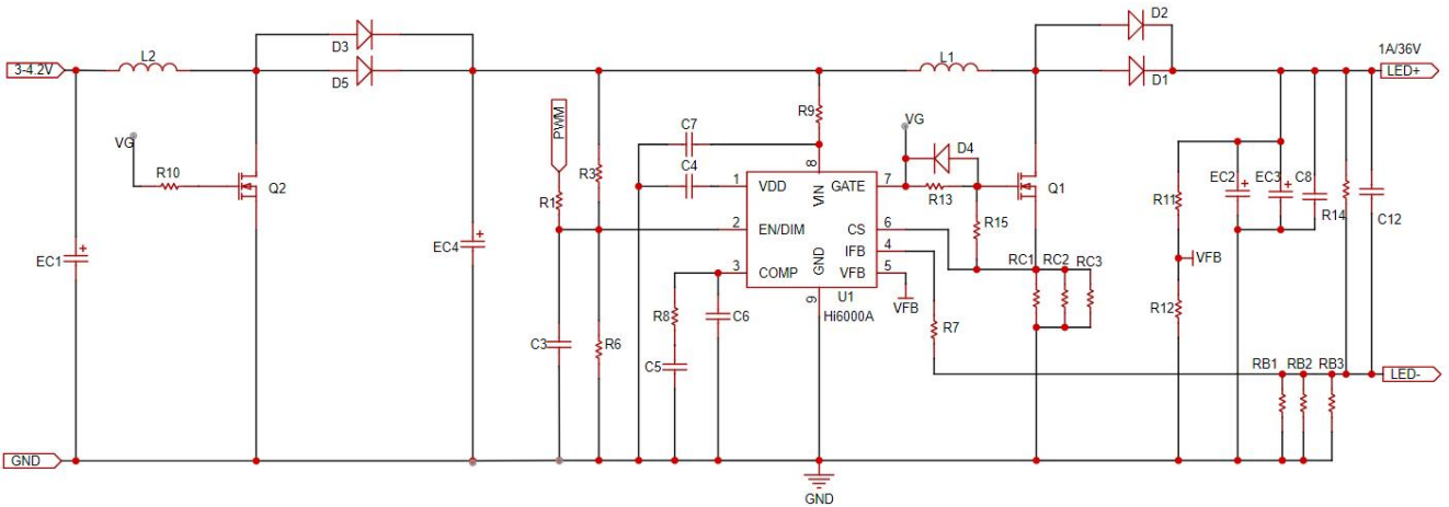
图 8.3 Hi6000A 两级升压应用电路
