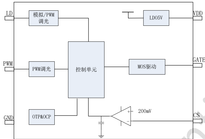
图 7-1 结构框图
