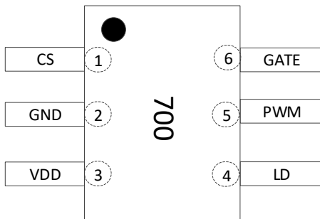
图 5-1 Hi7000D 管脚图
