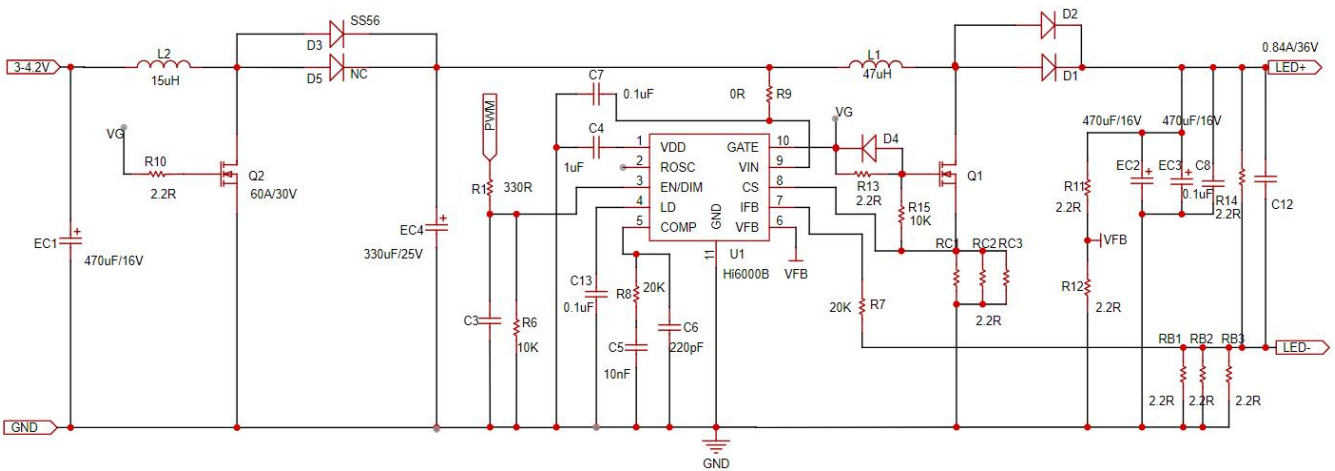
图 8.3 Hi6000B 两级升压应用电路
