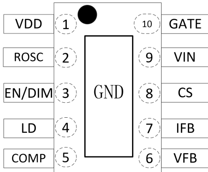
图 5.1 Hi6000B 管脚图
