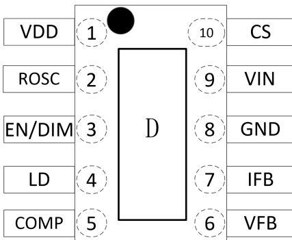
图 5.2 Hi6001 管脚图
