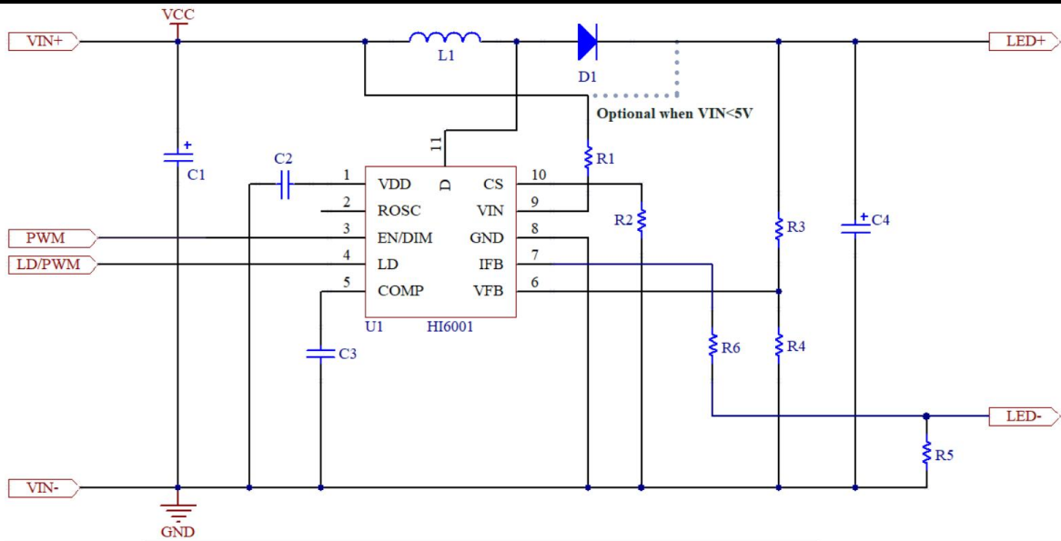
图 8.4 Hi6001 典型应用电路
