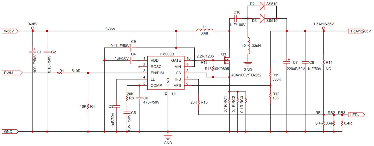
图 8.2 Hi6000B 升降压应用电路
