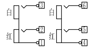
电原理图
