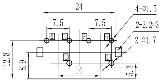
元件面孔位图
