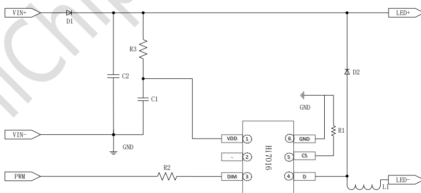
图 4.1 Hi7016 应用电路
