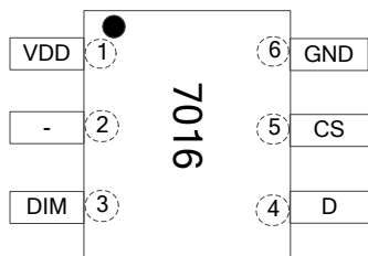
图 5.1 Hi7016 管脚图
