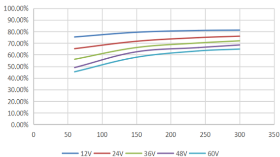
V_{OUT}=3.3V 效率图
