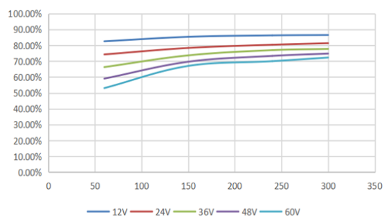
V_{OUT}=5V 效率图
