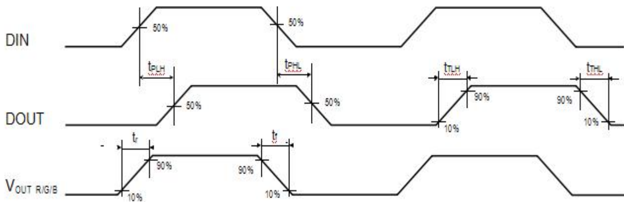
IC 动态参数测试示意图
