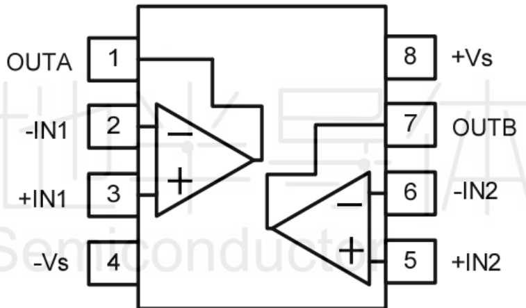
SOP8/DIP8/MSOP8/TSSOP8
