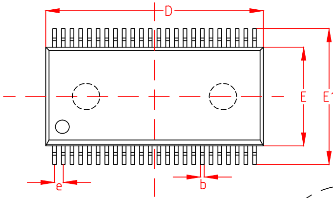
TOP VIEW 正视图
