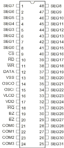
HT1621BRSZ SSOP48
