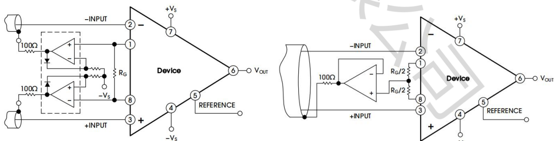
共模屏蔽驱动器
