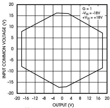
输入共模范围与输出电压, G = 1 (36V)
