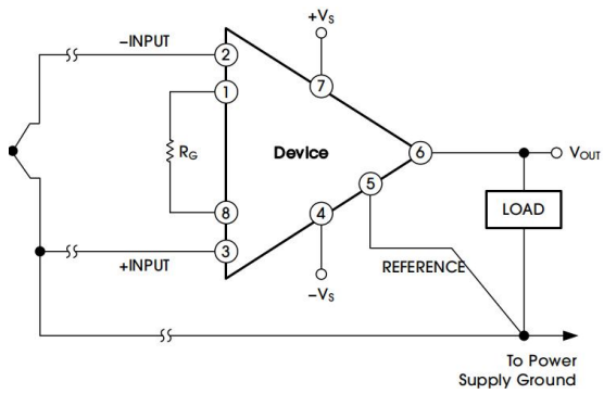
热电偶输入时的偏置电流接地回路
