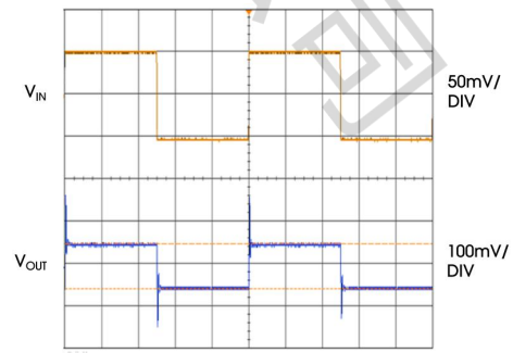
小信号响应 (G = 1)
