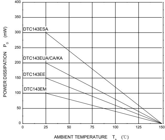
P_D — T_a
