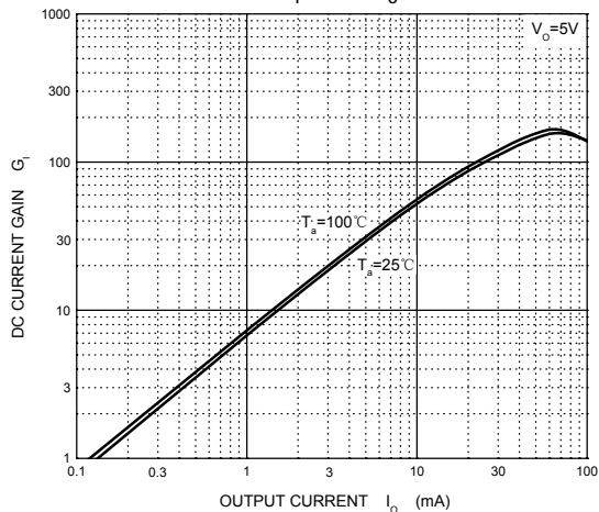
G_I — I_O
