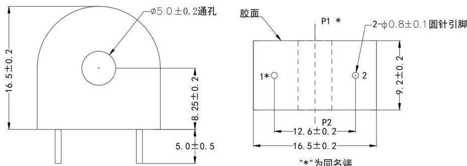
主视图
