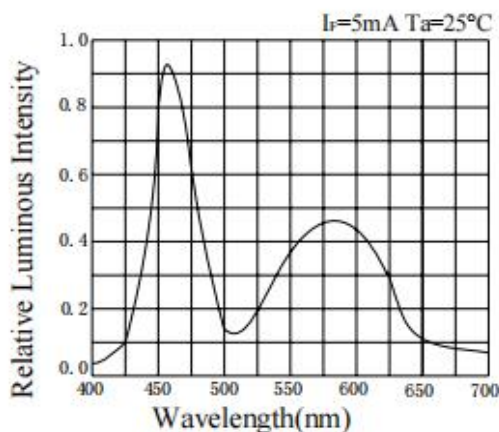
e) 相对光强—波长 e) RELATIVE INTENSITY VS. WAVELENGTH
