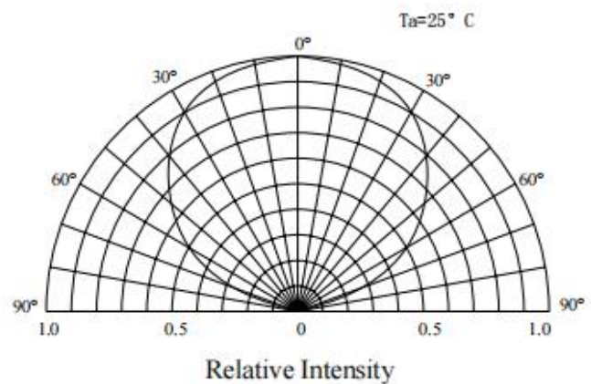
f) 辐射图 f) RADIATION PATTERN
