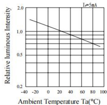
d) 相对光强—环境温度 d) RELATIVE INTENSITY VS. AMBIENT TEMPERATURE
