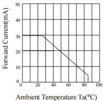
c) 正向电流—环境温度 c) FORWARD CURRENT VS. AMBIENT TEMPERATURE
