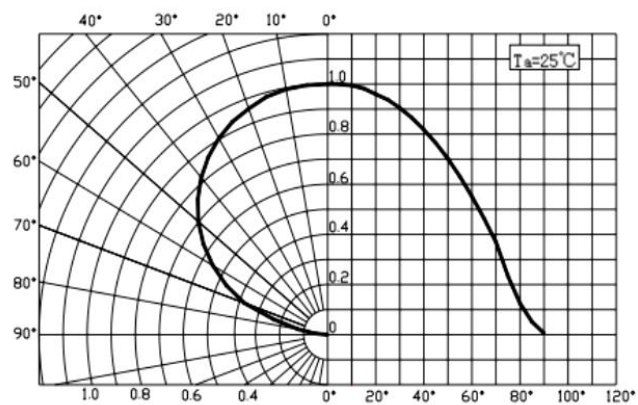
辐射特性曲线
