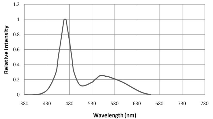
光谱分布特性曲线 Spectrum Distribution ( T_a=25^\circ\text{C} )
