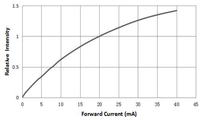
相对光强与电流特性曲线 Relative Intensity VS. Forward Current ( T_a=25^\circ\text{C} )
