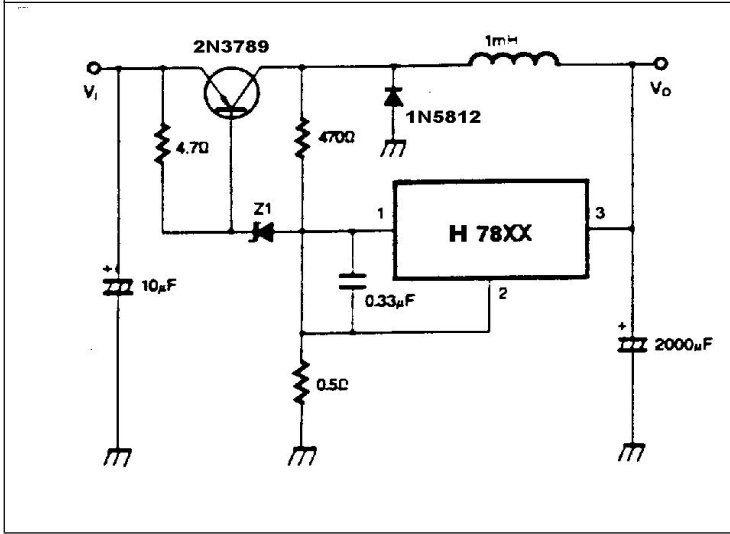
图13、开关稳压器
