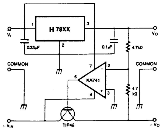
图 10、跟踪稳压器
