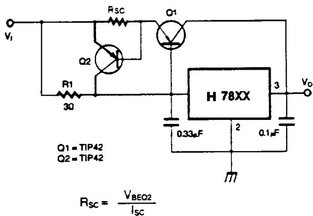
图 9、带短路保护的大电流输出
