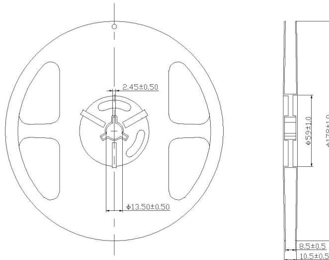
卷盘尺寸(单位:mm)
