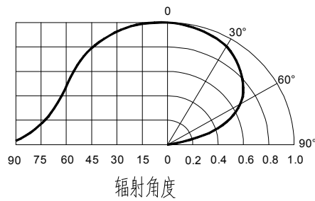
典型的辐射方向图 120°
