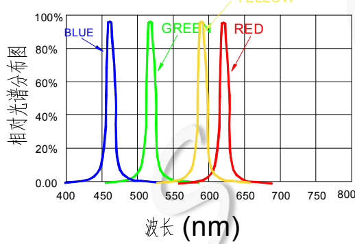
波长特性
