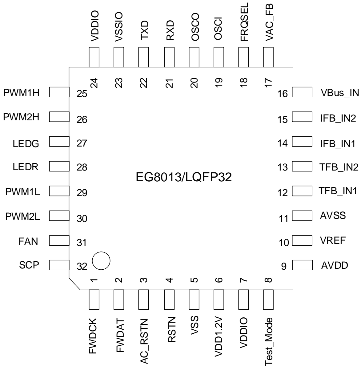
图 4-1. EG8013 管脚定义
