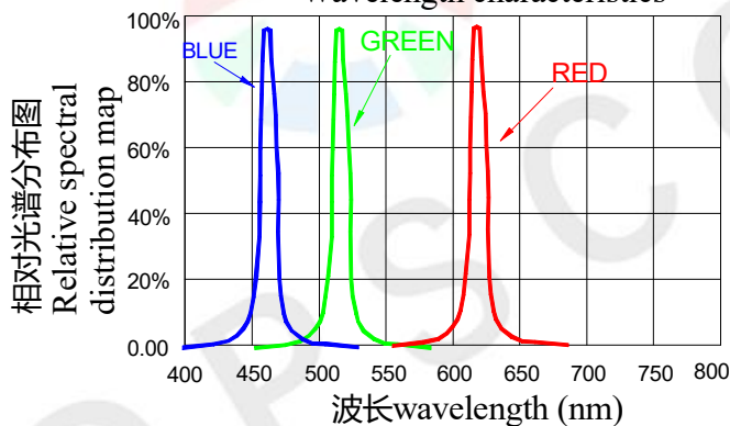
波长特性 Wavelength characteristics
