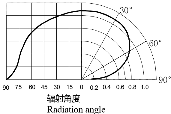
典型的辐射方向图 160° Typical radiation pattern 160°
