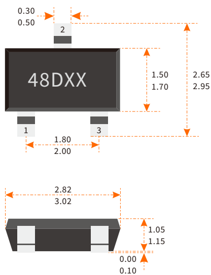
SOT-23 SO封装
