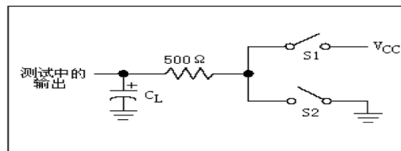
图 5:驱动器使能/无效定时测试负载
