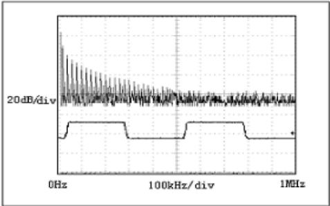
图11: 传输20kHz信号时 TDS3485EN-L/TR-TD 驱动器输出波形和FFT图
