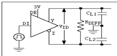
图 4:驱动器定时测试负载
