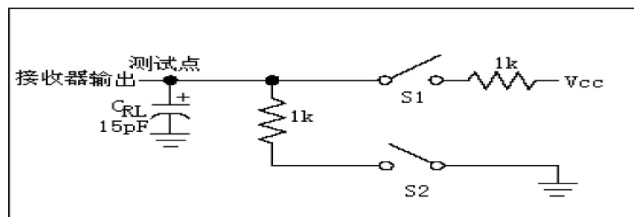
图 3:接收器使能/无效定时测试负载
