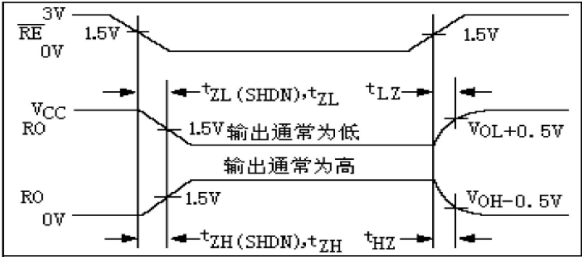
图 9:接收器使能和无效时间
