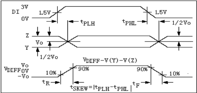
图 6:驱动器传播延时
