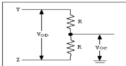
图 2:驱动器 DC 测试负载
