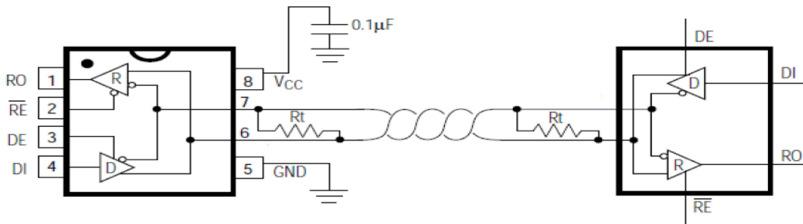
图 1：TDS3485EN-L/TR-TD 典型半双工应用电路
