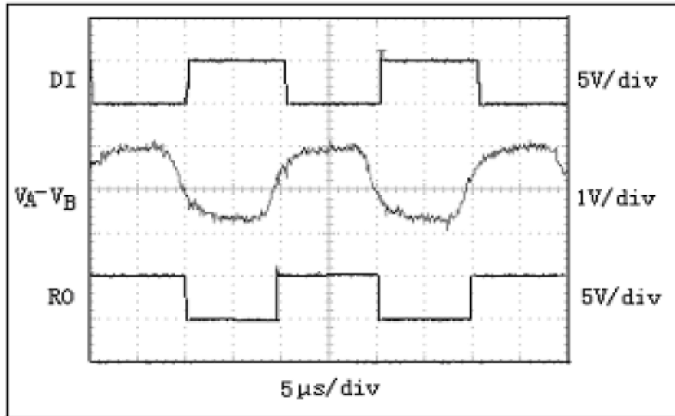
图 12: 在 50kHz 时驱动 4000 英尺的电缆
