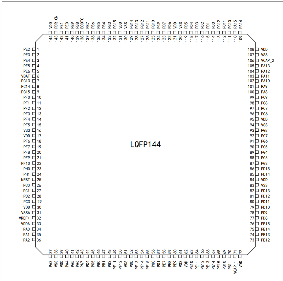
图2 TDS32F407VET6TR-TD系列LQFP144引脚分布图
