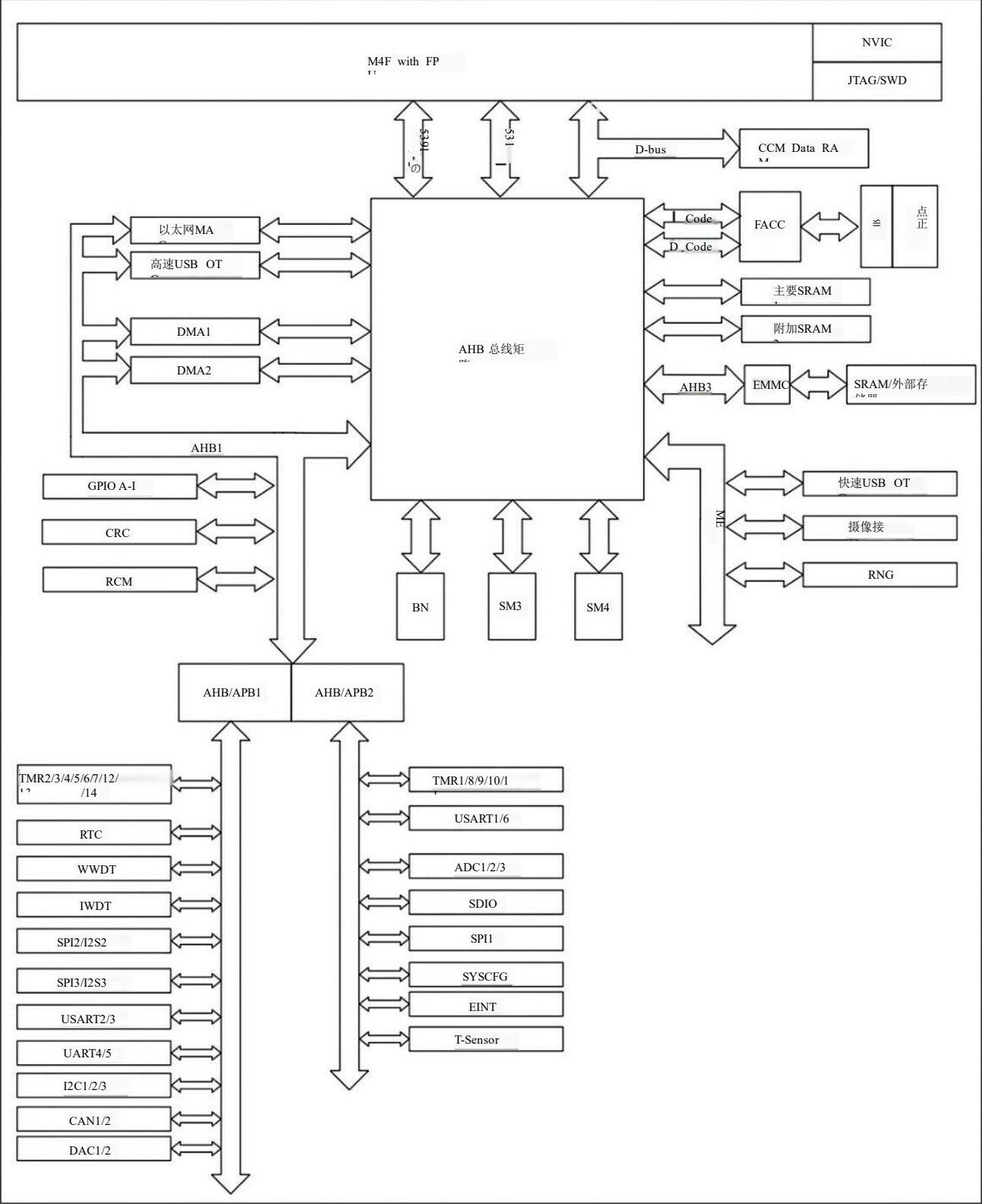
图 6 TDS32F407VET6TR-TD系统框图
