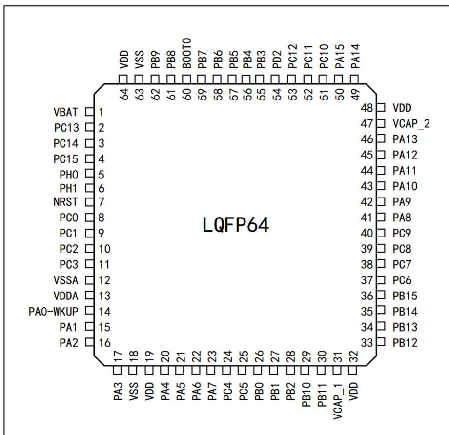
图 4 TDS32F407VET6TR-TD系列 LQFP64引脚分布图
