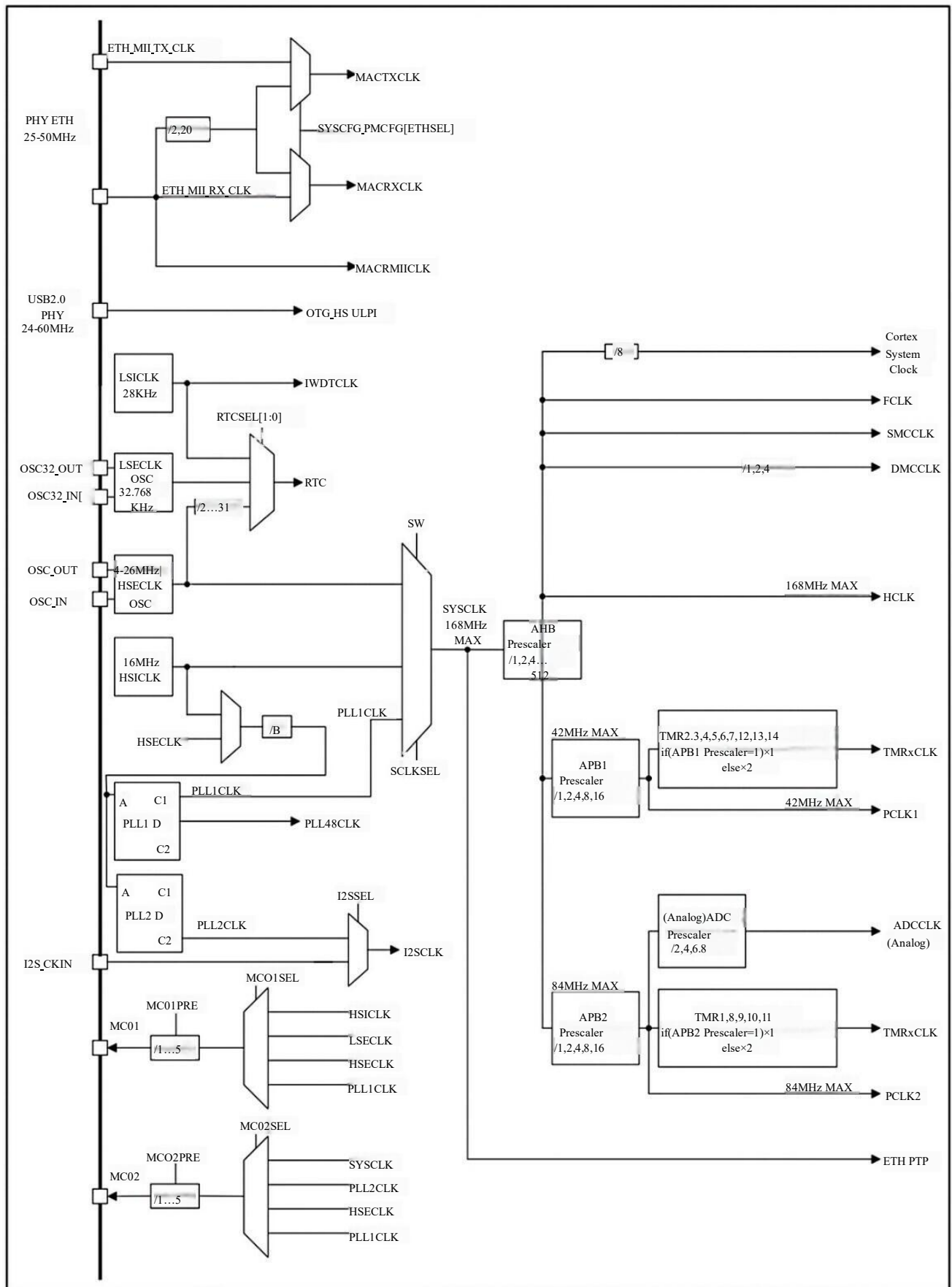
图 7 TDS32F407VET6TR-TD时钟树
