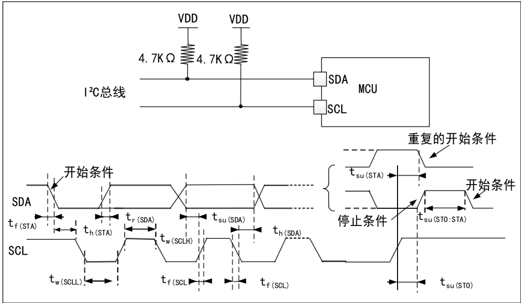
总线交流波形和测量电路
