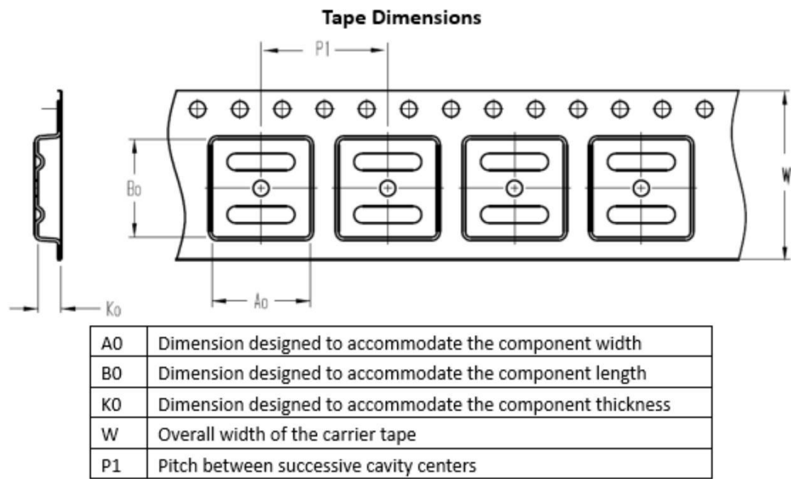
带状包装规格图
