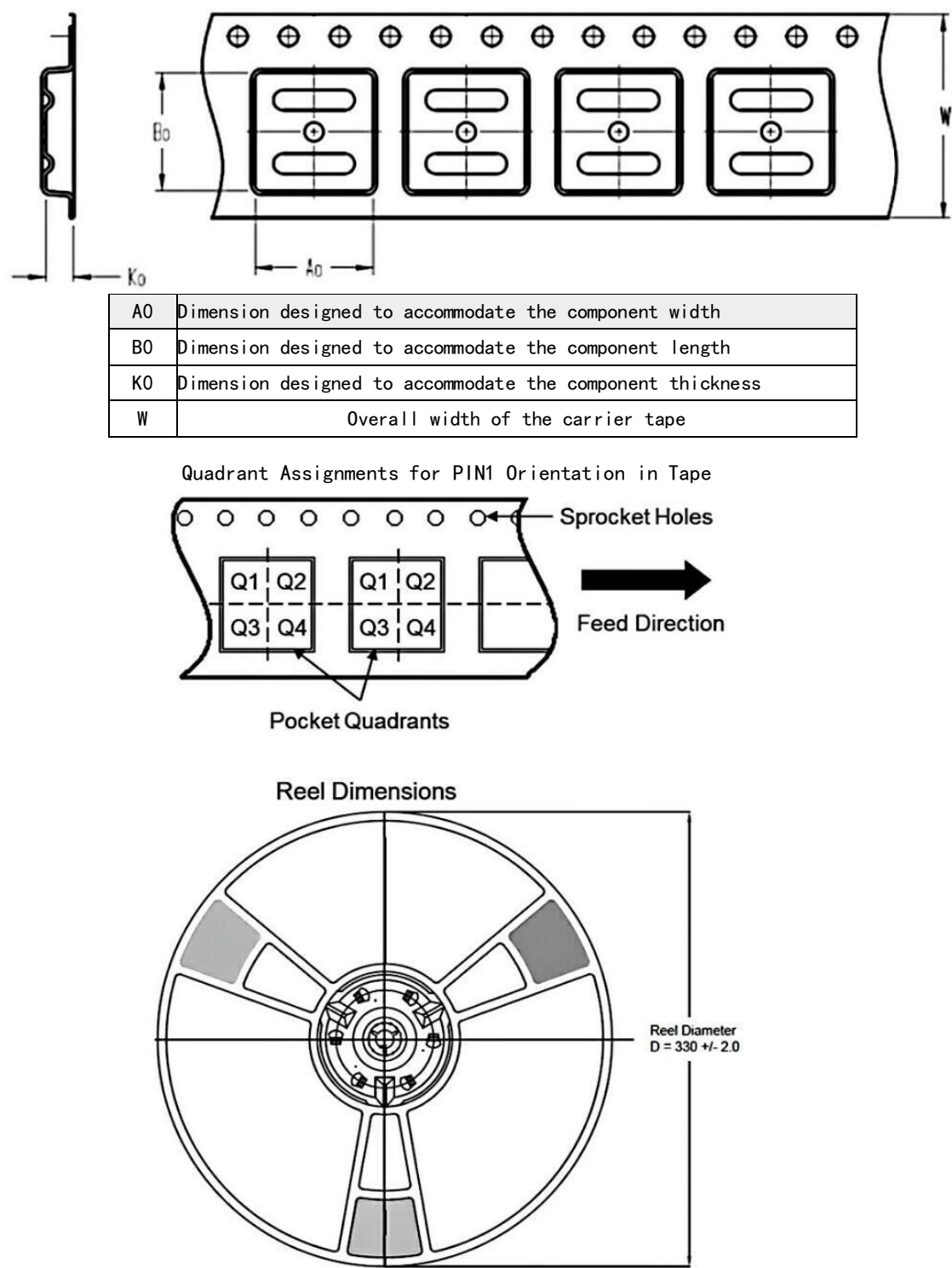
图 2 7 带状包装规格图
