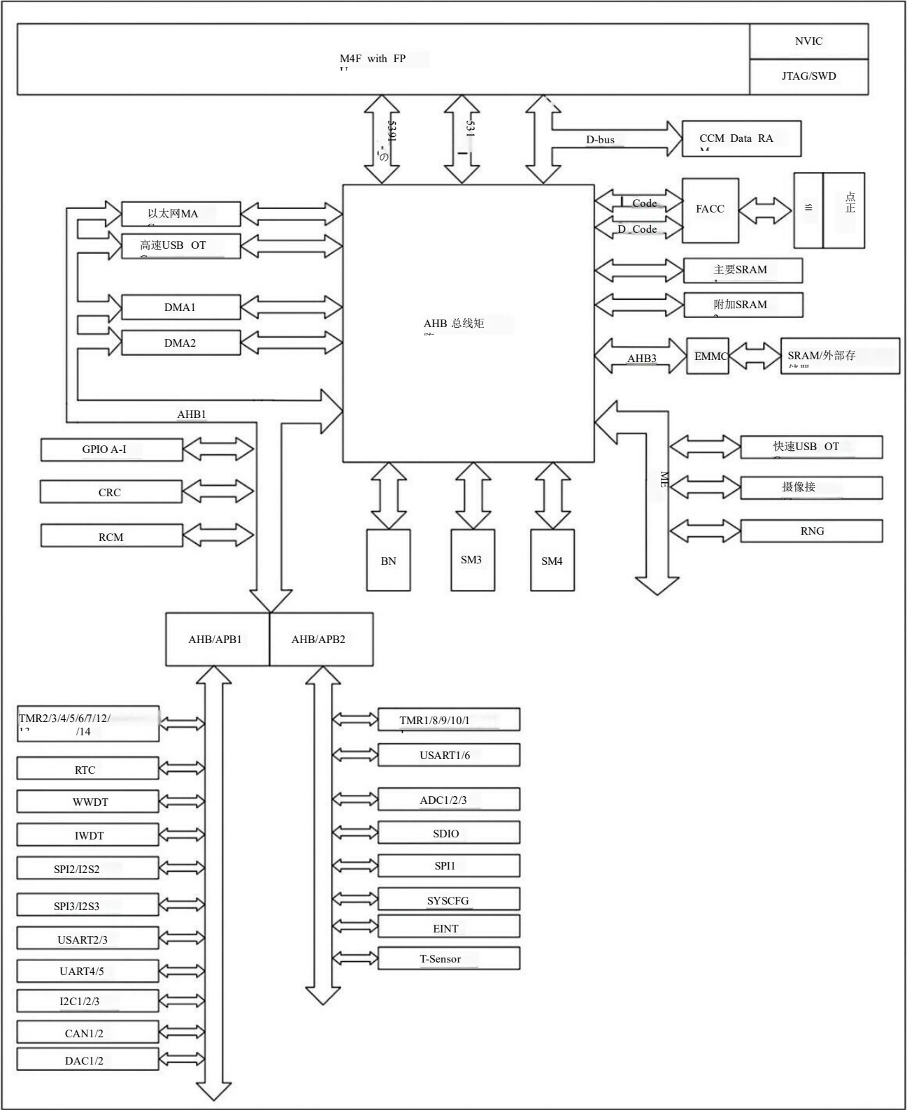
图 6 TDS32F407RGT6-TD系统框图
