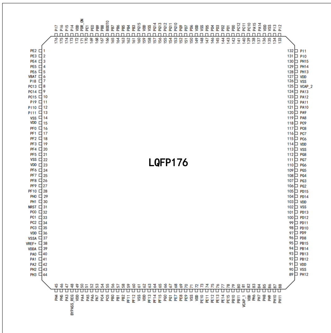
图 1 TDS32F407RGT6-TD 系列 LQFP176引脚分布图
