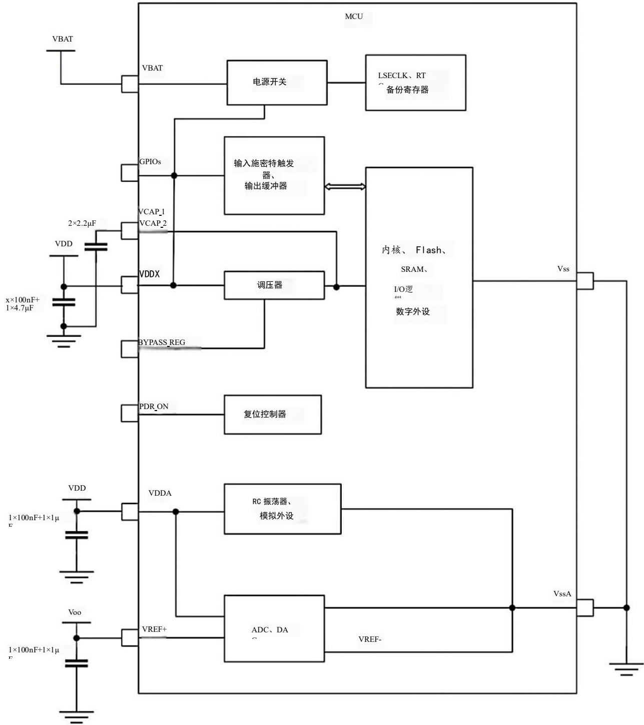
图 8 电源方案
