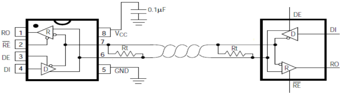
图 1: TDS485EEN-L/TR-TD 典型半双工应用电路
