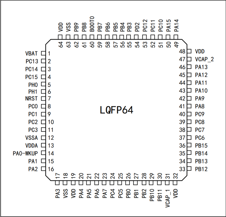
图 4 TDS32F407ZGT6-TD 系列 LQFP64 引脚分布图
