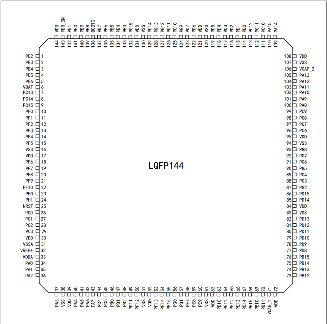
图2 TDS32F407ZGT6-TD 系列LQFP144引脚分布图
