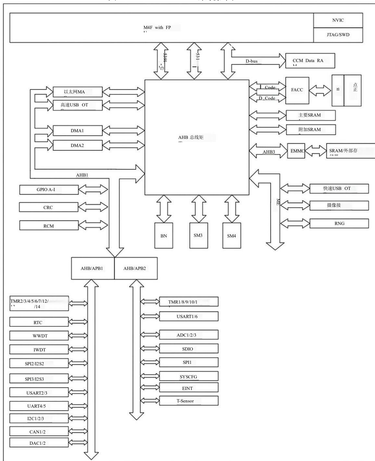
图 6 TDS32F407ZGT6-TD系统框图
