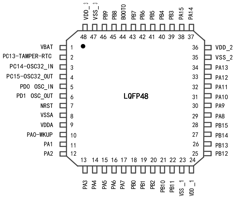
引脚分布图
