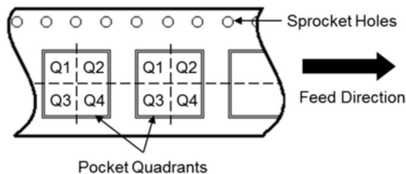
Reel Dimensions
